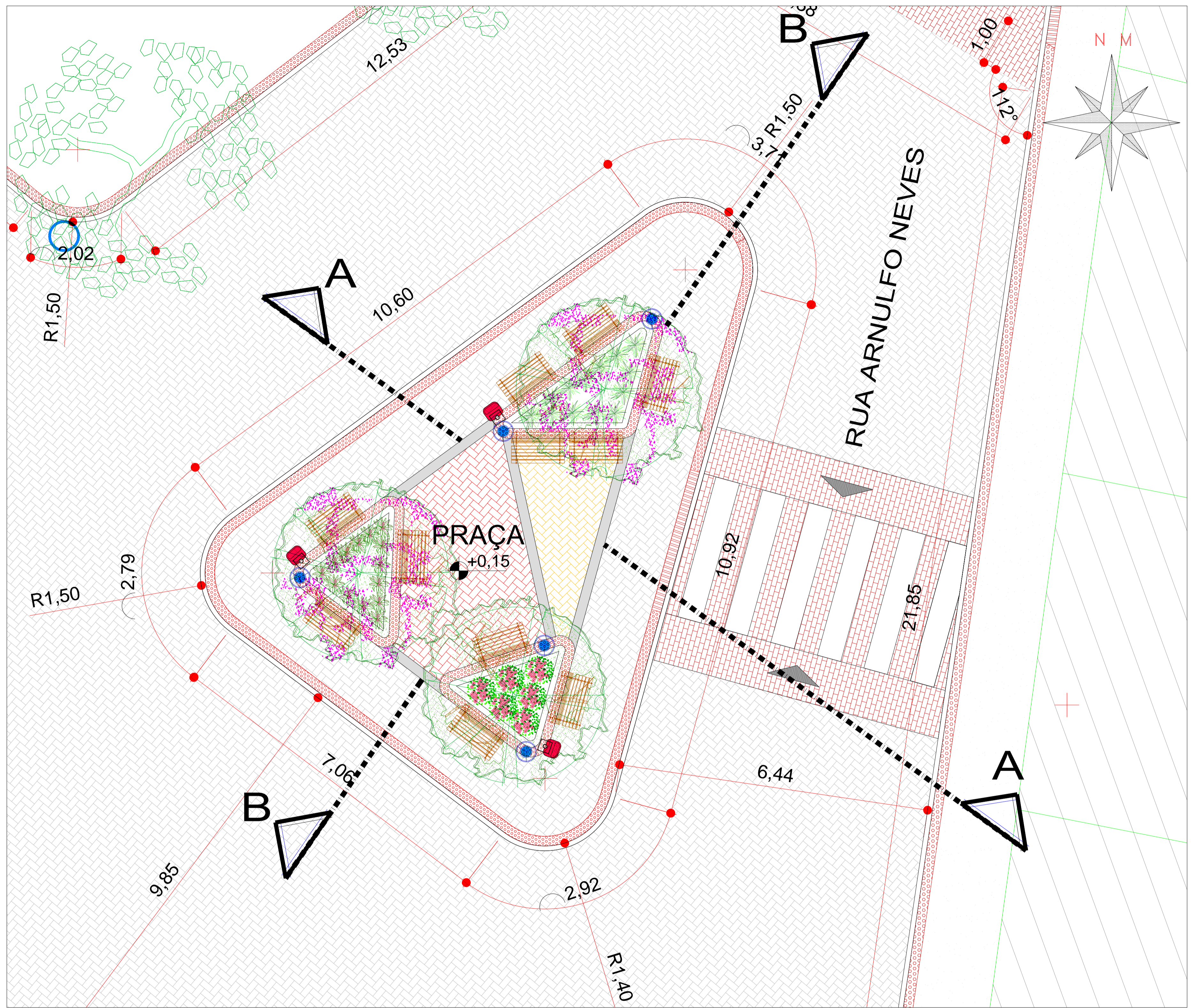
PLANTA BAIXA - PRAÇA ESCALA 1:50
