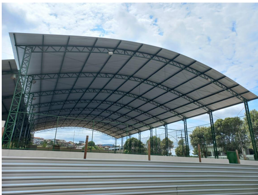
Foto 02: Cobertura nova em telha metálica
